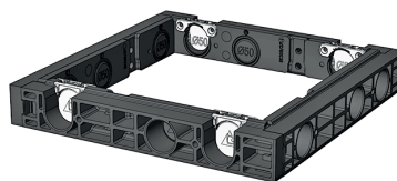
Rahmen 70 mm überbaubar Art.-Nr.: 06 358 0358E 2 x überbaubar / 1 x Ø 50 3 x Ø 50 Gewicht: 3,2 kg
