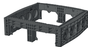
Rahmen 220 mm überbaubar Art.-Nr.: 06 388 0073E 2 x Rechteck 4 x Ø 110 Gewicht: 17,0 kg
