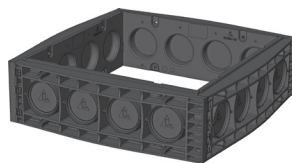
Rahmen 220 mm überbaubar Art.-Nr.: 06 388 0052E 4 x Ø 110 4 x Ø 110 Gewicht: 19,0 kg
