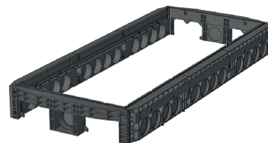
Rahmen 220 mm überbaubar Art.-Nr.: 06 738 0061E 2 x Rechteck / 1 x Ø 110 12 x Ø 110 Gewicht: 57,0 kg
