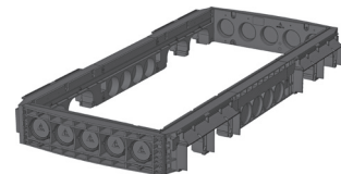
Rahmen 220 mm überbaubar Art.-Nr.: 06 738 0085E 5 x Ø 110 4 x Rechteck / 4 x Ø 110 Gewicht: 65,5 kg
