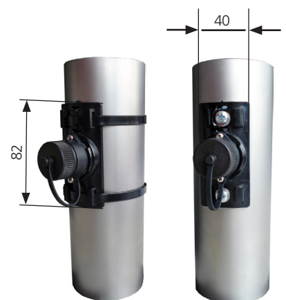
Befestigung am runden Mast mit Kabelbinder oder angeschraubt
